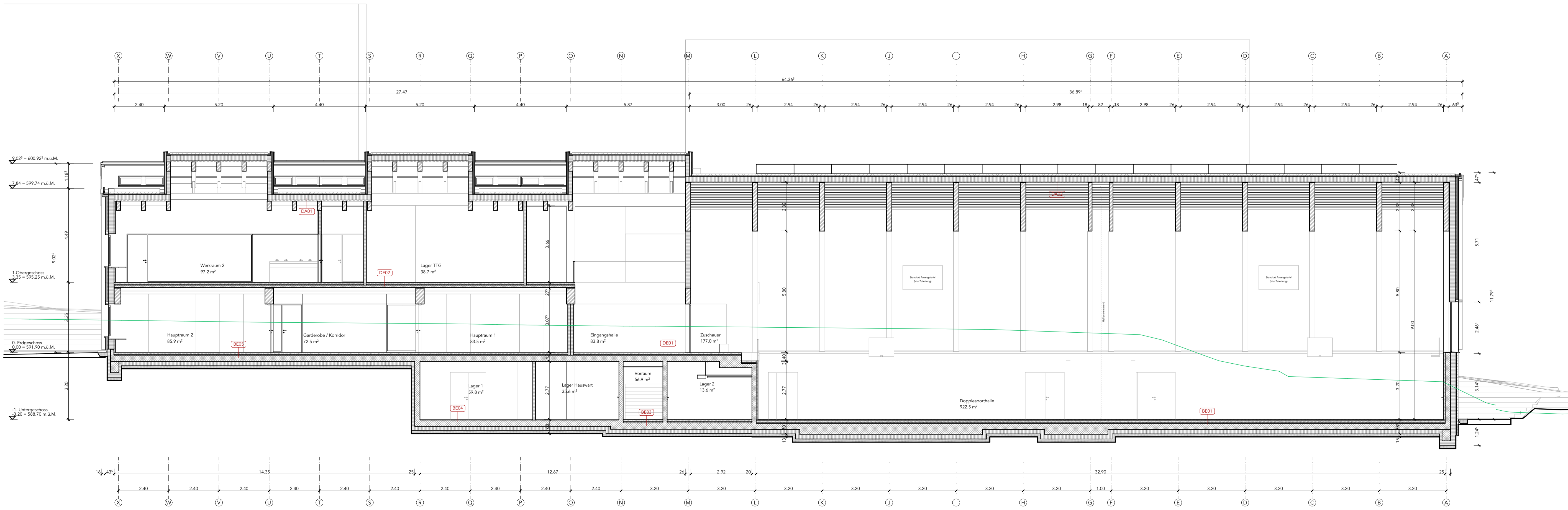
Schnitt 05
